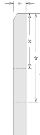
DOOR PROFILE BASE
